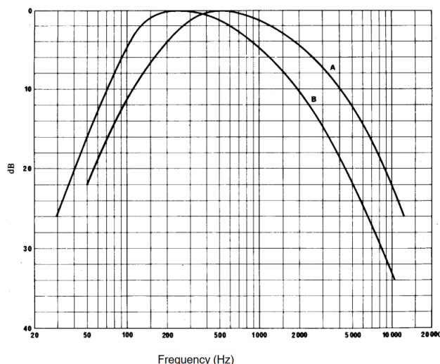
Figura B.1. Distribución espectral de la señal de prueba (Fuente: ETSI EN 300 422-1, 2021-11).
