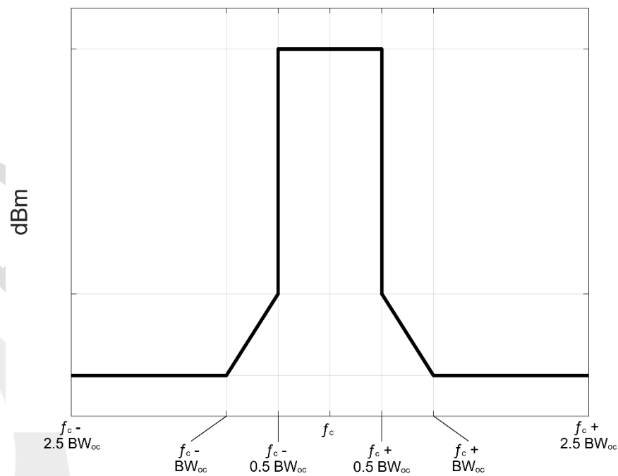
Figura C.5. Contorno de las Emisiones fuera de banda para WMA5.
