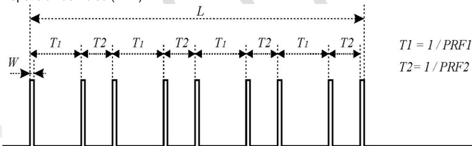
Figura 2C. Estructura general de la señal de prueba de radar de una sola ráfaga/ basada en un solo Pulso con PRF escalonado
