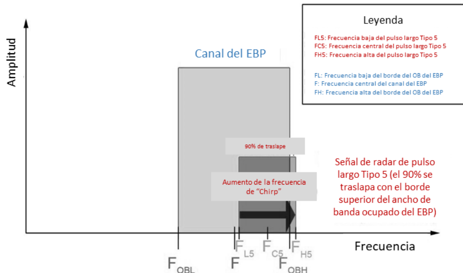
Figura 32. Ejemplo de la relación entre la señal de Pulso largo tipo 5 y el Canal WAS/RLAN cuando la señal está sintonizada de modo que el 90% de la señal de radar se superpone con el borde alto del Ancho de banda ocupado por EBP.
