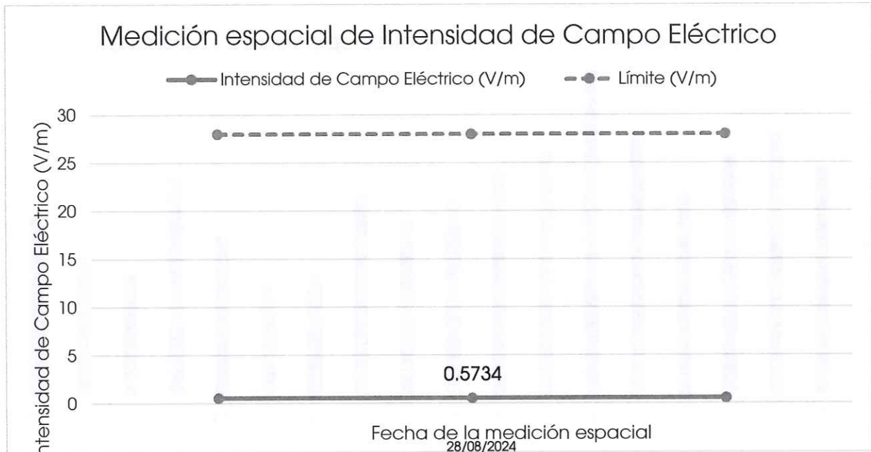
Imagen 7. Comparativo entre el valor espacial obtenido en el punto de medición 10 y el límite para campo eléctrico 28 V/m para exposición poblacional.
