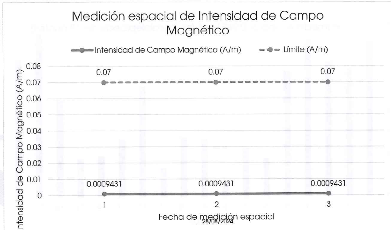
Imagen 8. Comparativo entre el valor espacial obtenido en el punto de medición 10 y el límite para campo magnético 0.073 A/m para exposición poblacional.
