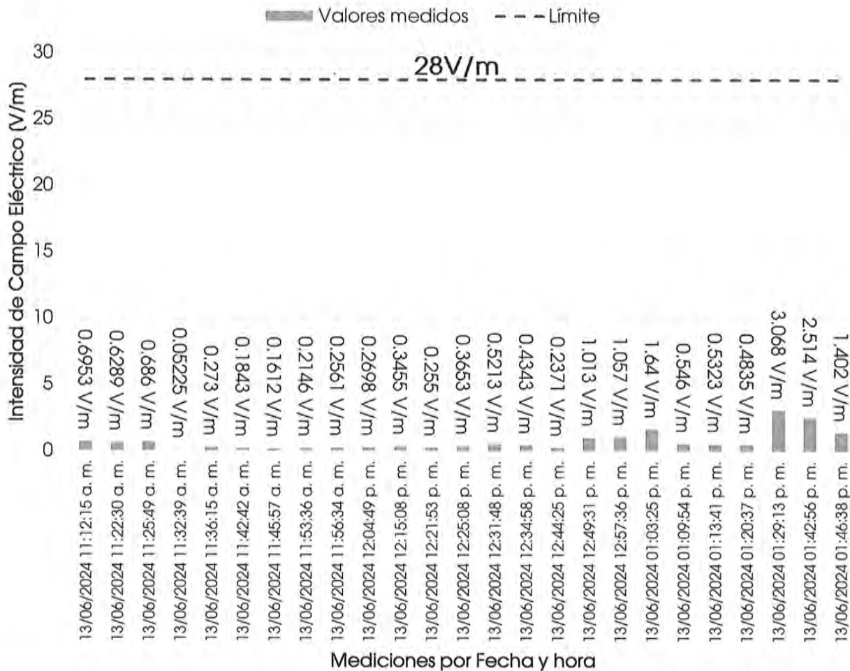
Imagen 4. Comparativo entre el valor promedio obtenido de cada punto indicado en la Tabla 3 y el límite de campo eléctrico de 28 V/m para exposición poblacional.
