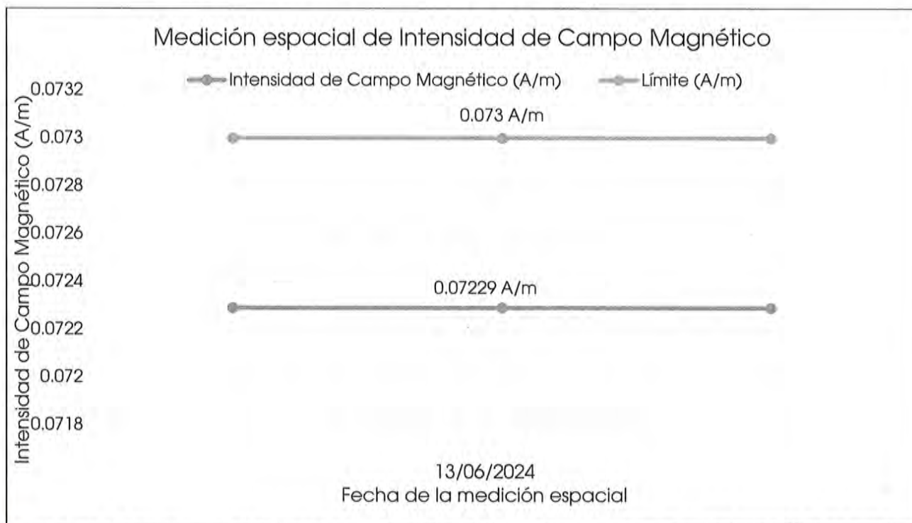
Imagen 8. Comparativo entre el valor espacial obtenido en el punto de medición 23 y el límite para campo magnético 0.073 A/m para exposición poblacional.
