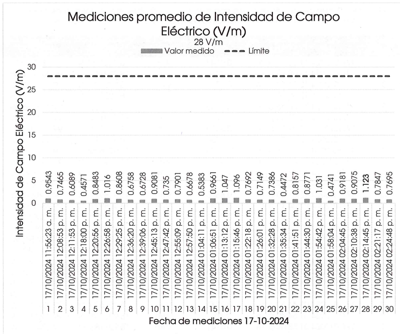
Imagen 4. Comparativo entre el valor promedio obtenido de cada punto indicado en la Tabla 4 y el límite de campo eléctrico de 28 V/m para exposición poblacional.
