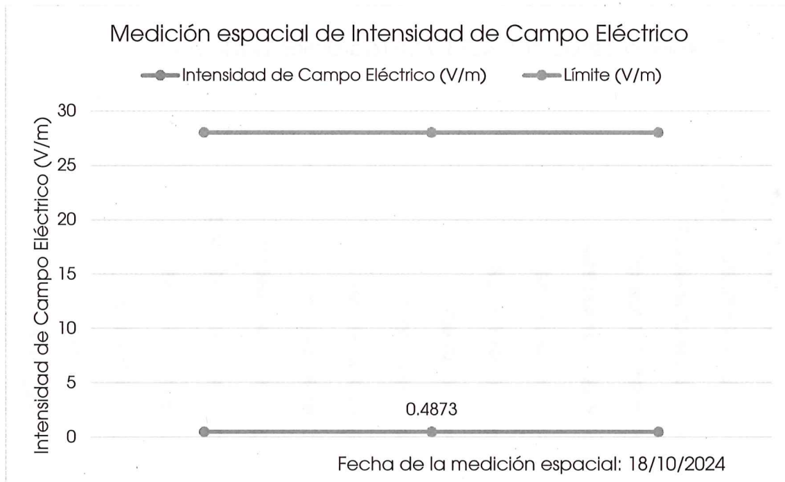
Imagen 7. Comparativo entre el valor espacial obtenido en el punto de medición 28 y el límite para campo eléctrico 28 V/m para exposición poblacional.
