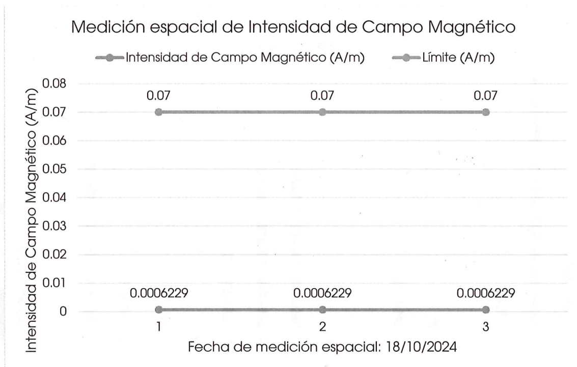
Imagen 8. Comparativo entre el valor espacial obtenido en el punto de medición 28 y el límite para campo magnético 0.073 A/m para exposición poblacional.
