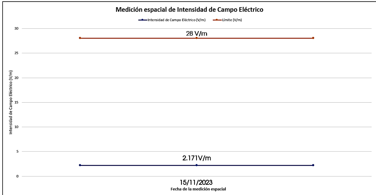
Imagen 20. Comparativo entre el valor espacial obtenido en el punto de medición 12 y el límite para campo eléctrico 28 V/m para exposición poblacional.
