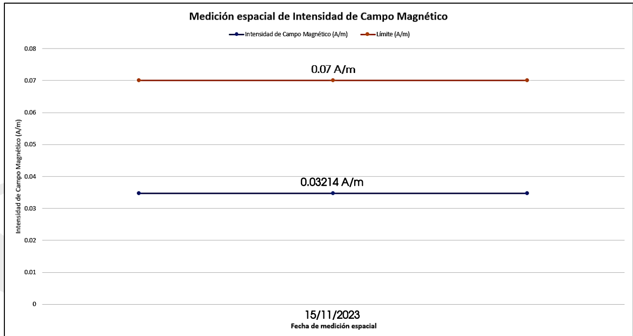
Imagen 21. Comparativo entre el valor espacial obtenido en el punto de medición 12 y el límite para campo magnético 0.073 A/m para exposición poblacional.
