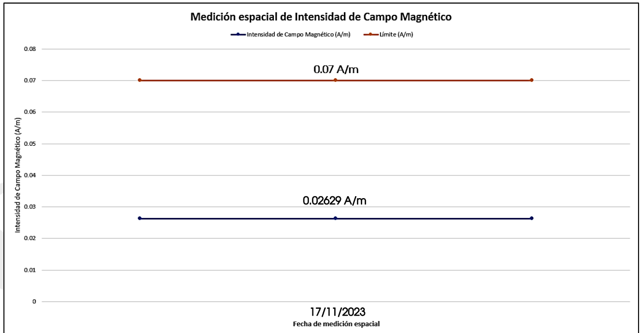
Imagen 28. Comparativo entre el valor espacial obtenido en el punto de medición 19 y el límite para campo magnético 0.073 A/m para exposición poblacional.
