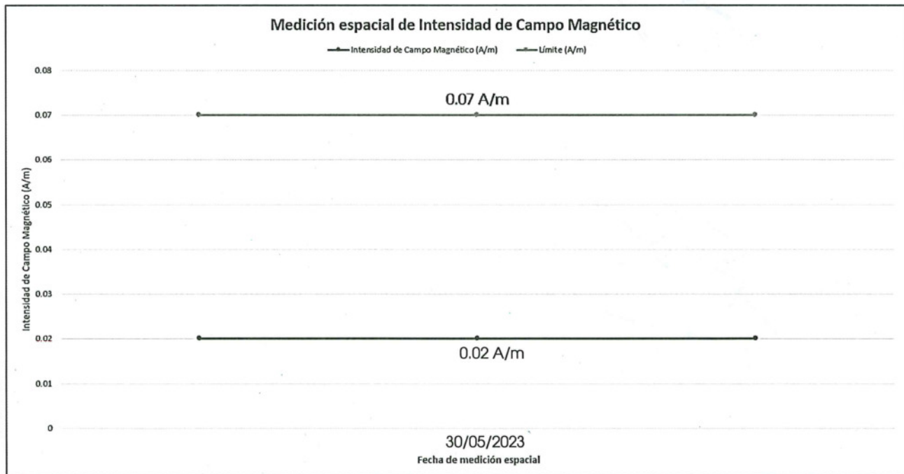
Imagen 32. Comparativo entre el valor espacial obtenido en el exterior del domicilio donde habita la denunciante y el límite para campo magnético 0.073 A/m para exposición poblacional.
