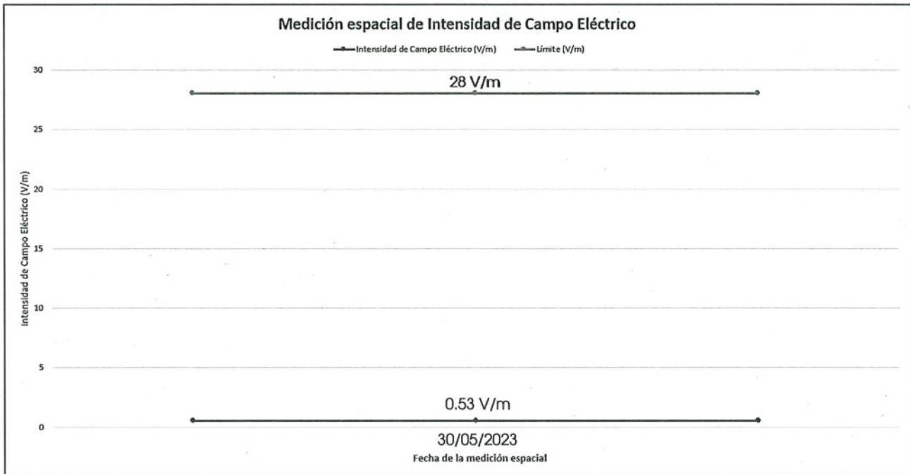
Imagen 31. Comparativo entre el valor espacial obtenido en el exterior del domicilio donde habita la denunciante y el límite para campo eléctrico 28 V/m para exposición poblacional.
