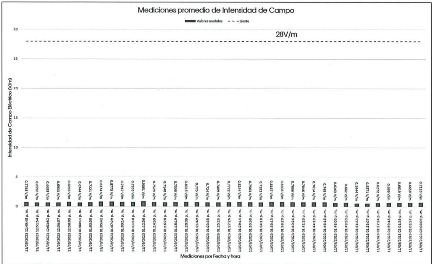
Imagen 4. Comparativo entre el valor promedio obtenido de cada punto indicado en la Tabla 3 y el límite de campo eléctrico de 28 V/m para exposición poblacional.
