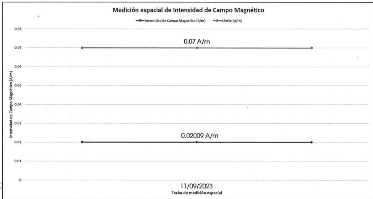
Imagen 46. Comparativo entre el valor espacial obtenido en el punto de medición 12 y el límite para campo magnético 0.073 A/m para exposición poblacional.
