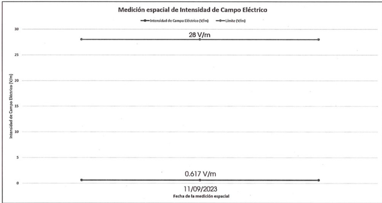
Imagen 45. Comparativo entre el valor espacial obtenido en el punto de medición 12 y el límite para campo eléctrico 28 V/m para exposición poblacional.
