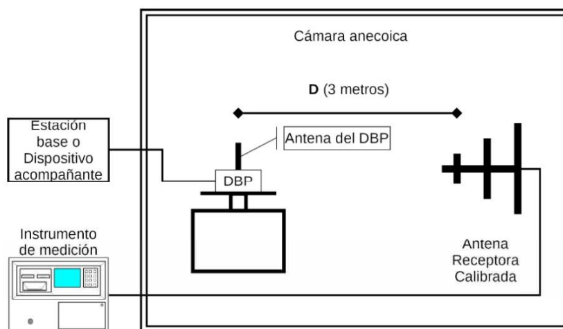
Figura 2. Configuración para medición de Emisiones radiadas.
