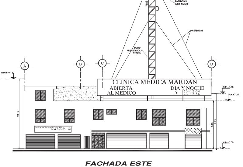
FACHADA ESTE
