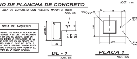
DL-1 ACOT. cm
