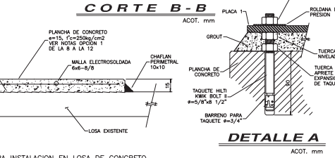
CORTE B-B ACOT. mm
