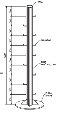
MASTIL SUPERIOR SUSTITUTO DE TRAMO T-45
