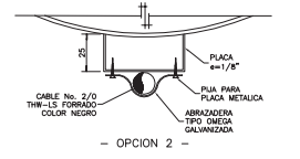
DETALLE DE SUJECION PARA CABLE DE PARARRAYOS
