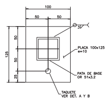
PLACA 1
