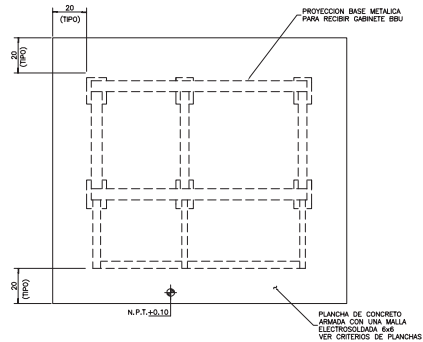
PLANCHA PARA BASE METALICA ACOT. cm
