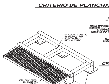
ISOMETRICO BASE METALICA
