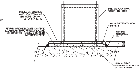
CORTE C-C
