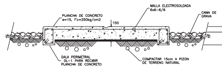
CRITERIO DE PLANCHA DE CONCRETO
