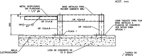
CORTE B-B ACOT. mm
