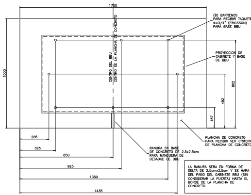
PLANCHA DE CONCRETO PARA BBU ACOT. mm
