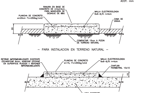
PLANCHA DE CONCRETO PARA BBU ACOT. mm
