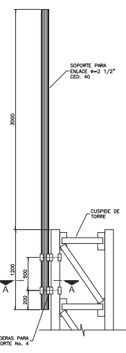
- DETALLE 2 -
