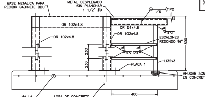
CORTE B-B
