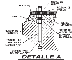
DETALLE A
