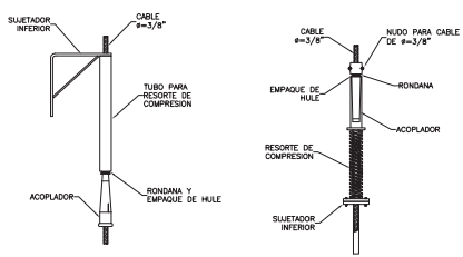
DETALLE A
