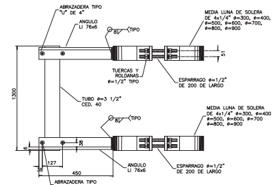
CORTE D-D
