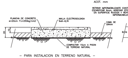
CORTE A-A ACOT. mm
