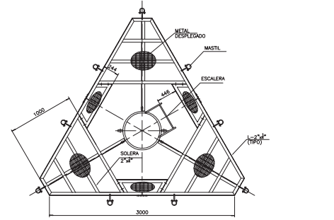
PLATAFORMA TRIANGULAR CELULAR DE 3m MARCO PARA PLATAFORMA
