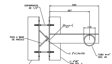
CORTE C-C
