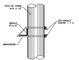
DETALLE 4
