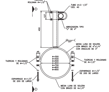
SOPORTE PARA MICROONDAS No. 8 (PARA MONOPOLOS DE \phi=300, 400, 500, 600, 700, 800 Y 900 mm)
