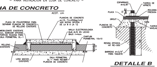
DETALLE B ACOT. mm
