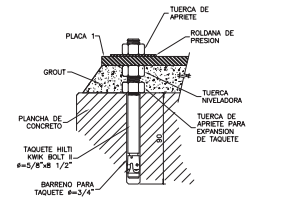
DETALLE A
