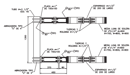
CORTE C-C
