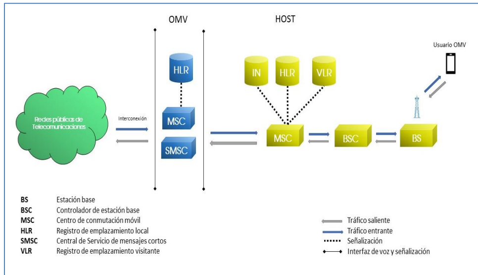
Diagrama 3. Flujo de tráfico de un OMV Completo/Agregador
