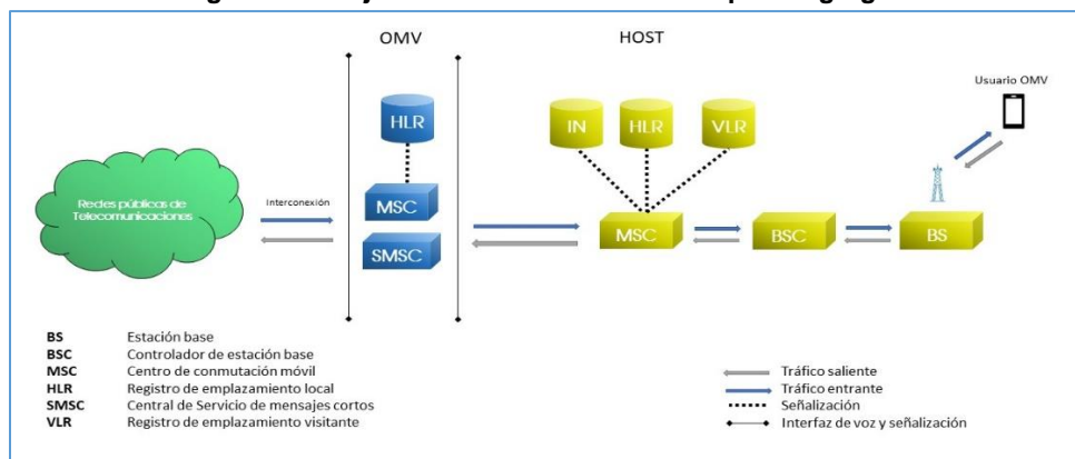
Diagrama 3. Flujo de tráfico de un OMV Completo/Agregador
