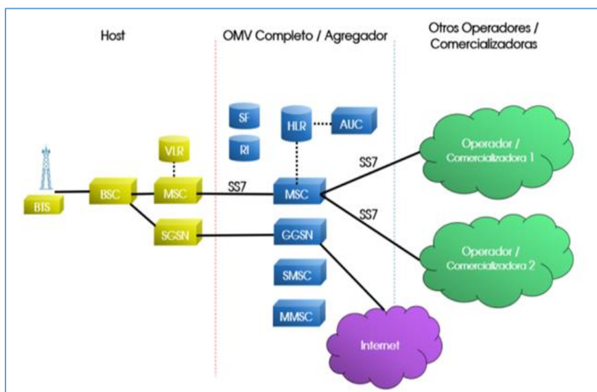
Diagrama 2. Elementos de la infraestructura de la red de un OMV Completo/Agregador
