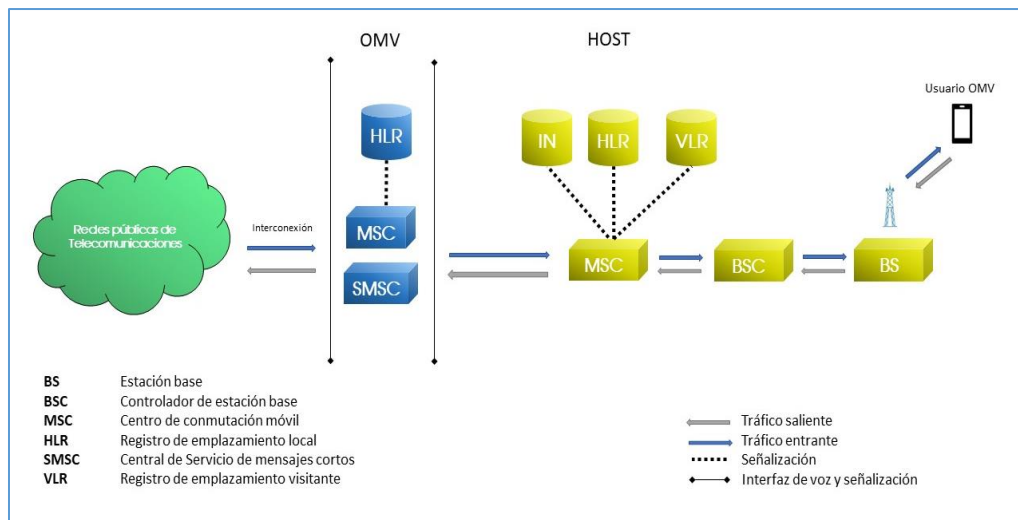
Diagrama 3. Flujo de tráfico de un OMV Completo/Agregador
