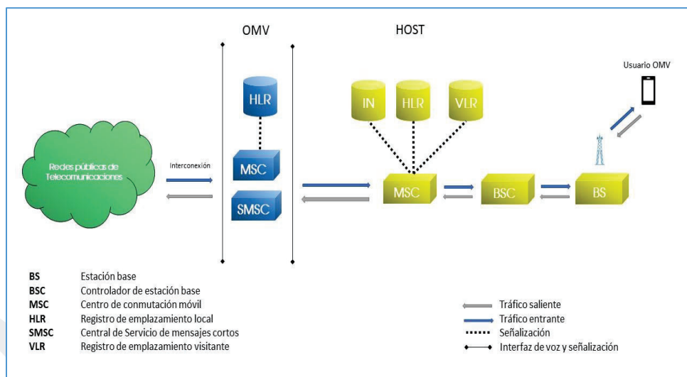
Diagrama 3. Flujo de tráfico de un OMV Completo/Agregador
