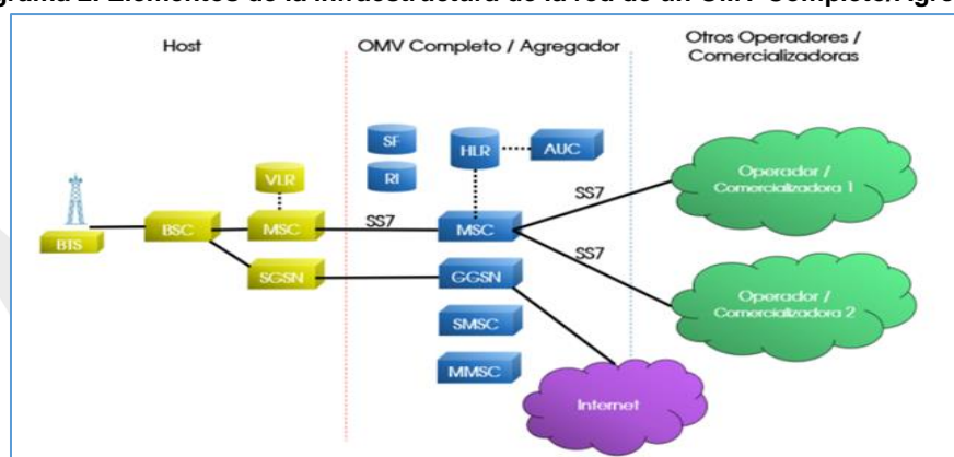
Diagrama 2. Elementos de la infraestructura de la red de un OMV Completo/Agregador
