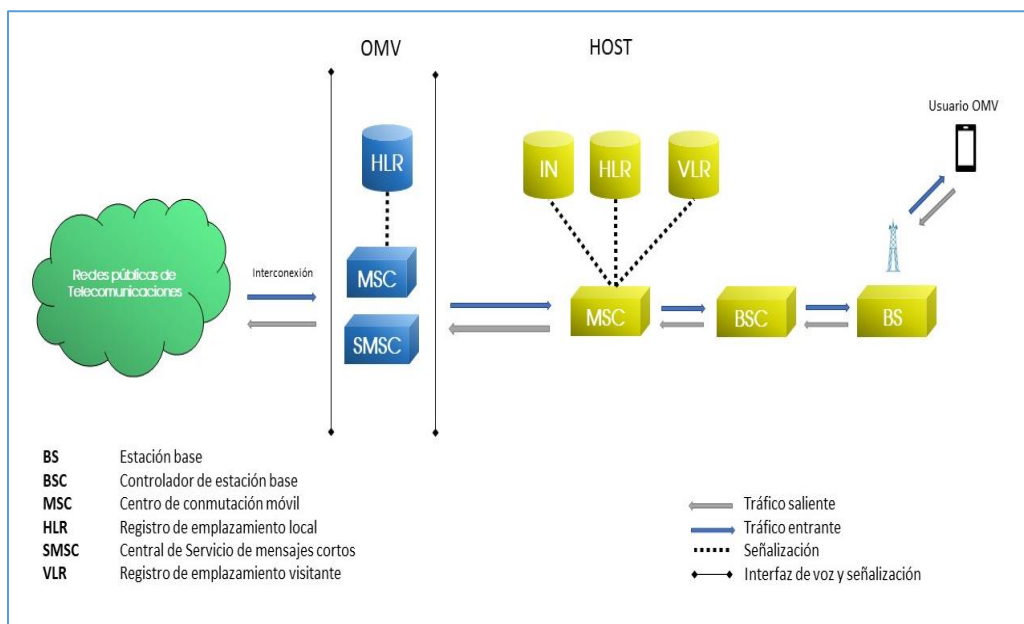
Diagrama 3. Flujo de tráfico de un OMV Completo/Agregador
