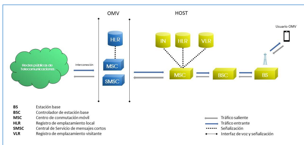
Diagrama 3. Flujo de tráfico de un OMV Completo/Aggregador
