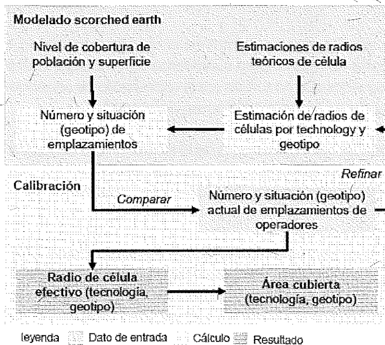
Figura 3: Esquema de modelado scorched earth calibrado para el operador móvil. (Fuente: Analysys Mason, 2012)
