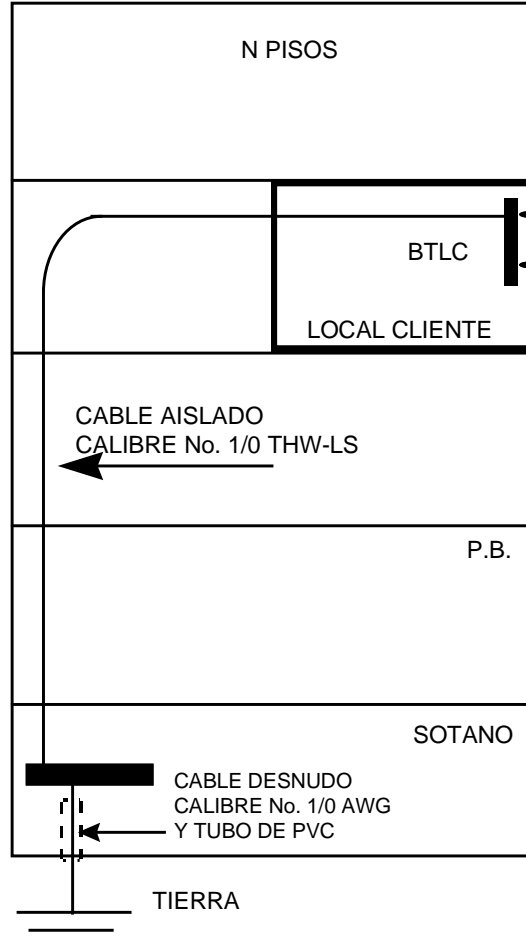
Puesta a Tierra del Local RDA Dentro de un Edificio Corporativo en un Piso Superior.
