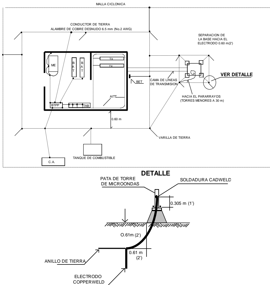
Torres Instaladas a Nivel de Piso.
