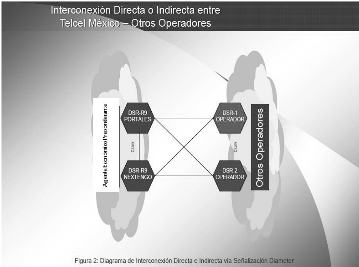
Figura 2: Diagrama de interconexión directa e indirecta vía señalización Diameter
